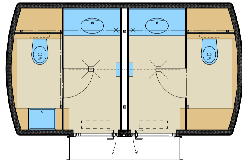
GRUNDRISS PARKREFUGIA 2 E29045PK 2
