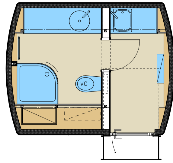
GRUNDRISS DOPPELSTANDART E29060DST
