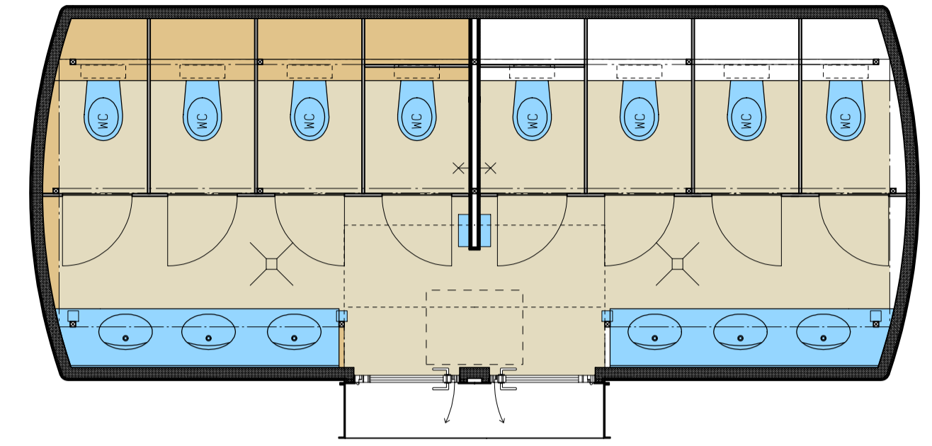
GRUNDRISS BEDÜRFNIS REFUGIA 2 DAMEN GROSS E35075BH2GRD
