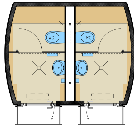
GRUNDRISS PARKREFUGIA 1 E29030PK 1
