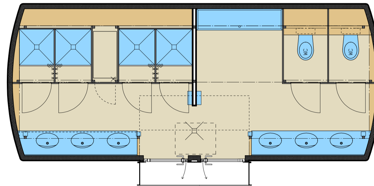
GRUNDRISS BEDÜRFNIS- & PFLEGE REFUGIA 2 HERREN E35075BPH2H
