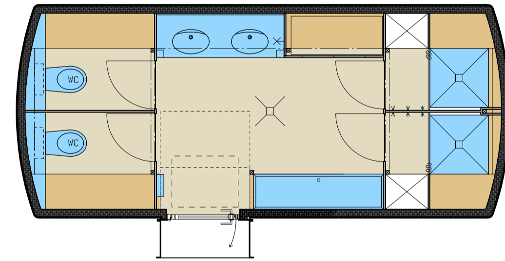
GRUNDRISS BEDÜRFNIS- & PFLEGEHÖHLE HERREN E29060BPH1H
