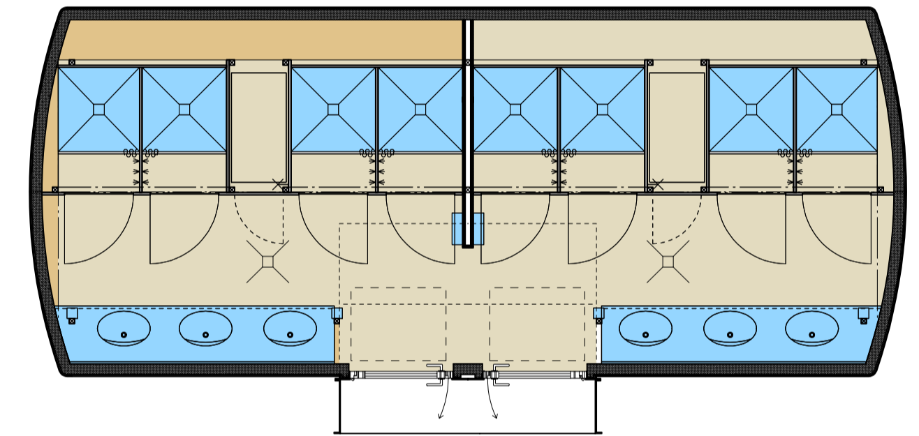
GRUNDRISS PFLEGE REFUGIA 2 GROSS DAMEN + HERREN E35075PH2GRD+H
