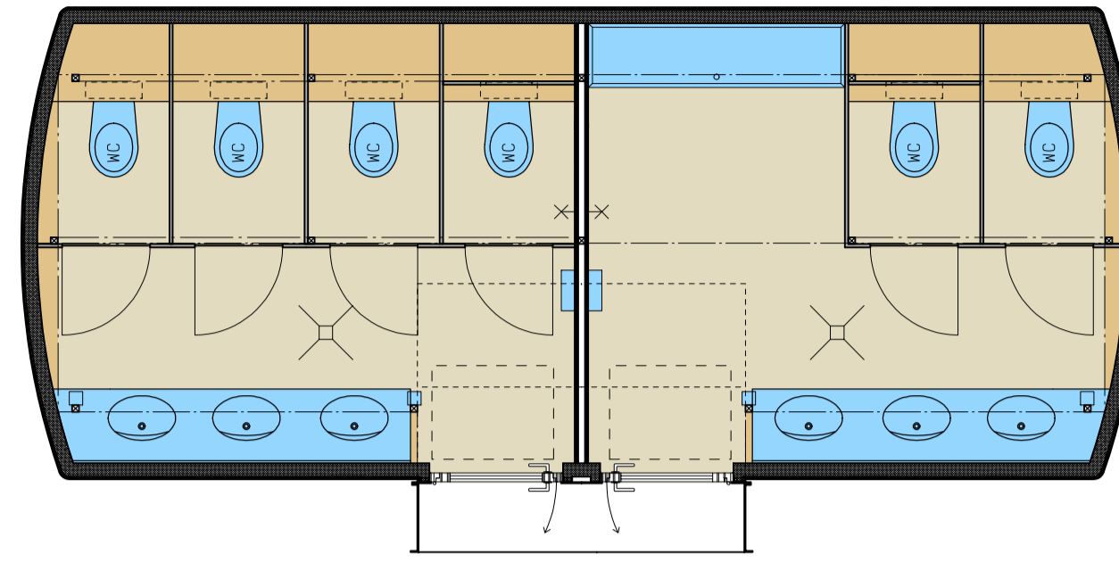
GRUNDRISS BEDÜRFNIS REFUGIA 2 E35075BH2
