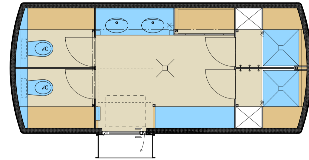
GRUNDRISS BEDÜRFNIS- & PFLEGE REFUGIA DAMEN E29060BPH1D
