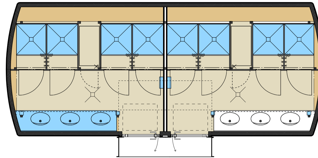
GRUNDRISS PFLEGE REFUGIA 2 E35075PH2
