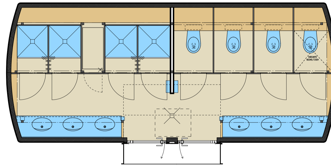
GRUNDRISS BEDÜRFNIS- & PFLEGE REFUGIA 2 DAMEN E35075BPH2D
