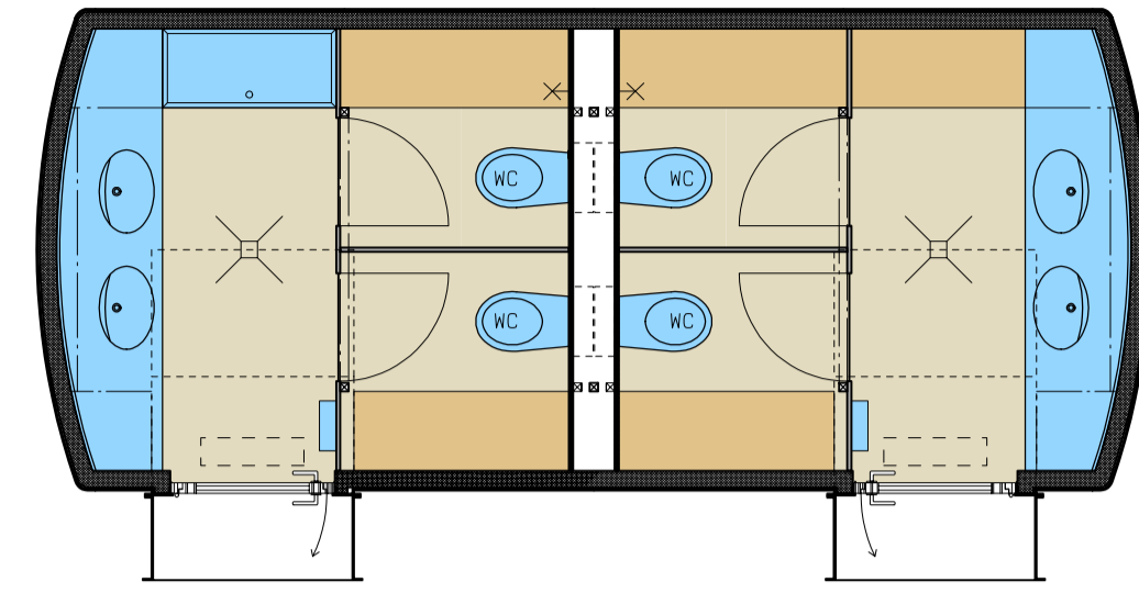
GRUNDRISS PFLEGE REFUGIA E29060PH1
