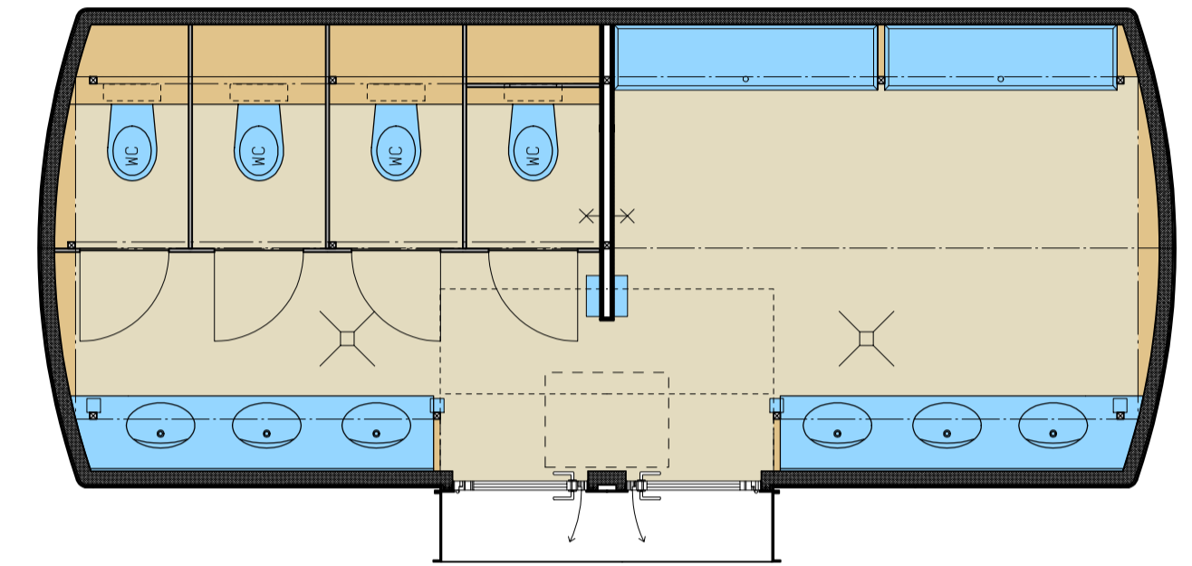
GRUNDRISS BEDÜRFNIS REFUGIA 2 HERREN GROSS E35075BH2GRH
