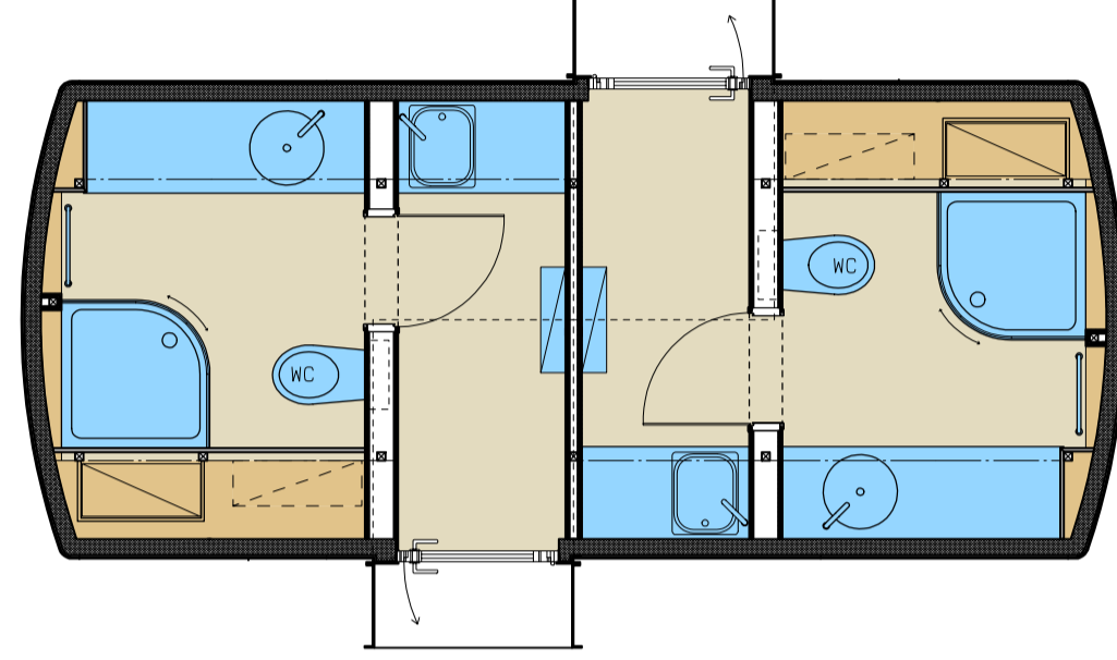
GRUNDRISS DOPPELSTANDART E29060DST
